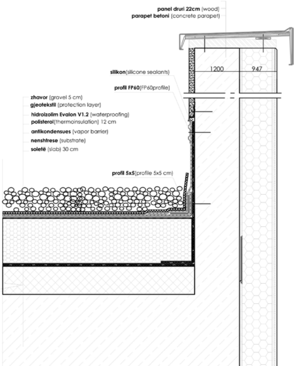
Detaj 3
