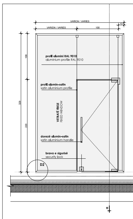
PAMJE VETRATË WINDOWS ELEVATION
