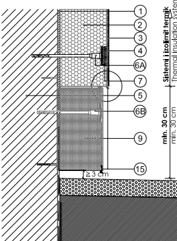
Detaj 3 (Varianti II) Detail 3 (Varianti II)
