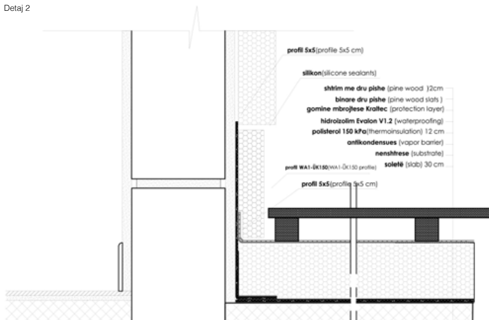
Detaj 2
