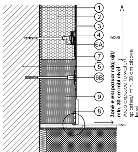
Detaj 1 Detail 1
