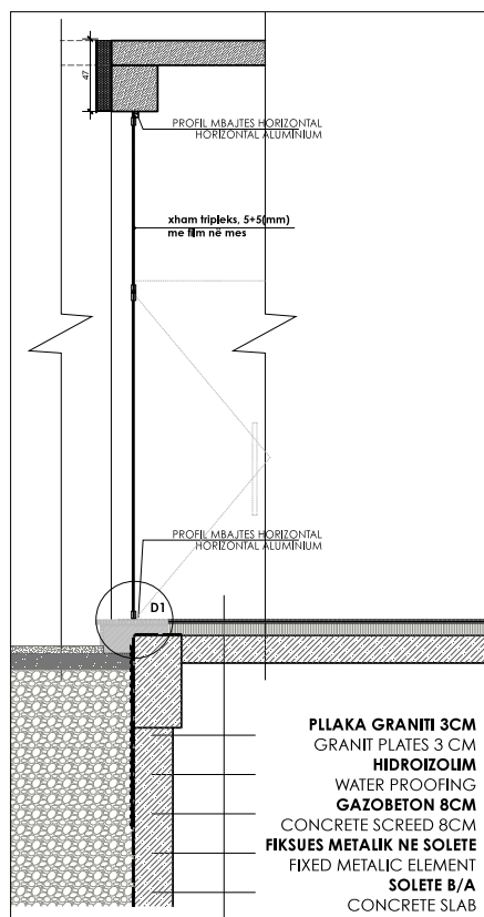
PRERJA A-A SH. 1:30 SECTION A-A SC. 1:30
