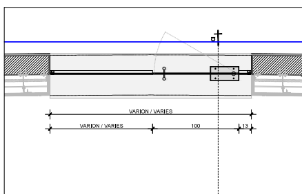
VETRATAT NË KATIN PRËDHE GROUND FLOOR WINDOWS
