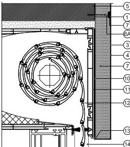
Detaj 2 Detail 2
