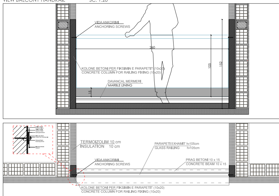
Pamje Kangjella ne llozha VIEW BALCONY HANDRAIL
